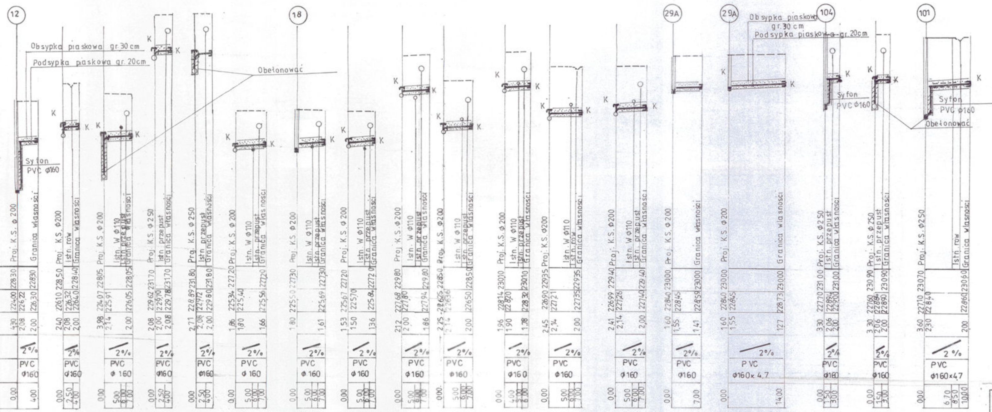
Profil podłużny przyłączy kanalizacji sanitarnej do granicy posesji w Babach Skala 1: 500/100
